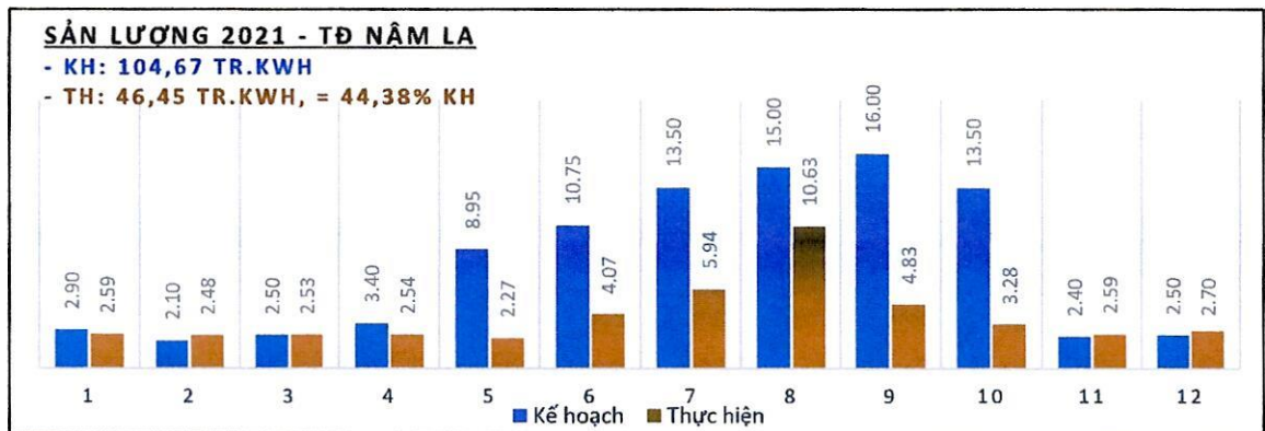
Biểu sản lượng 2021 của NMTĐ Nậm La (KH và TH hàng tháng)
