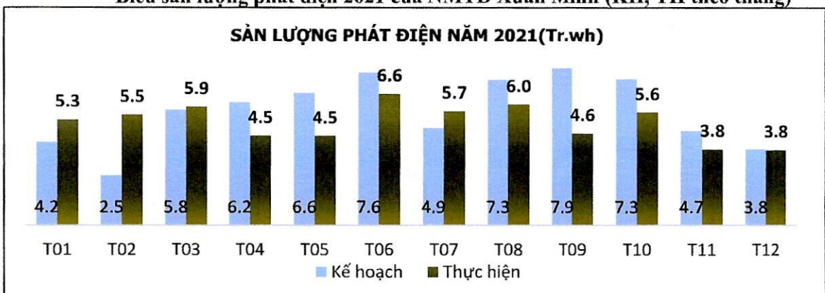
Biểu sản lượng phát điện 2021 của NMTĐ Xuân Minh (KH, TH theo tháng)
