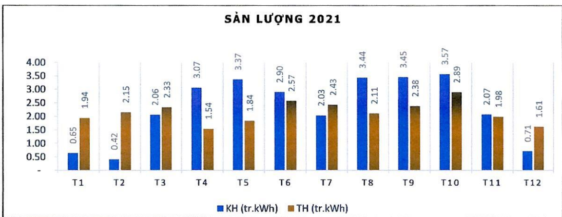
Biểu sản lượng phát điện năm 2021 của NMTĐ Bái Thượng
