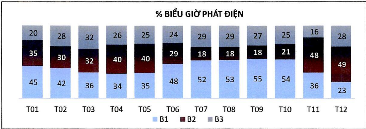
Biểu % giờ phát điện năm 2021 của NMTĐ Xuân Minh
