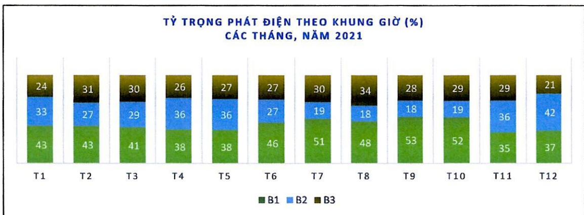
Biểu % giờ phát điện năm 2021 của NMTĐ Bái Thượng
