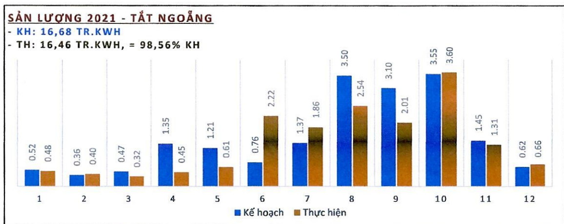
Biểu sản lượng 2021 của NMTĐ Tắt Ngoẵng (KH và TH hàng tháng)
