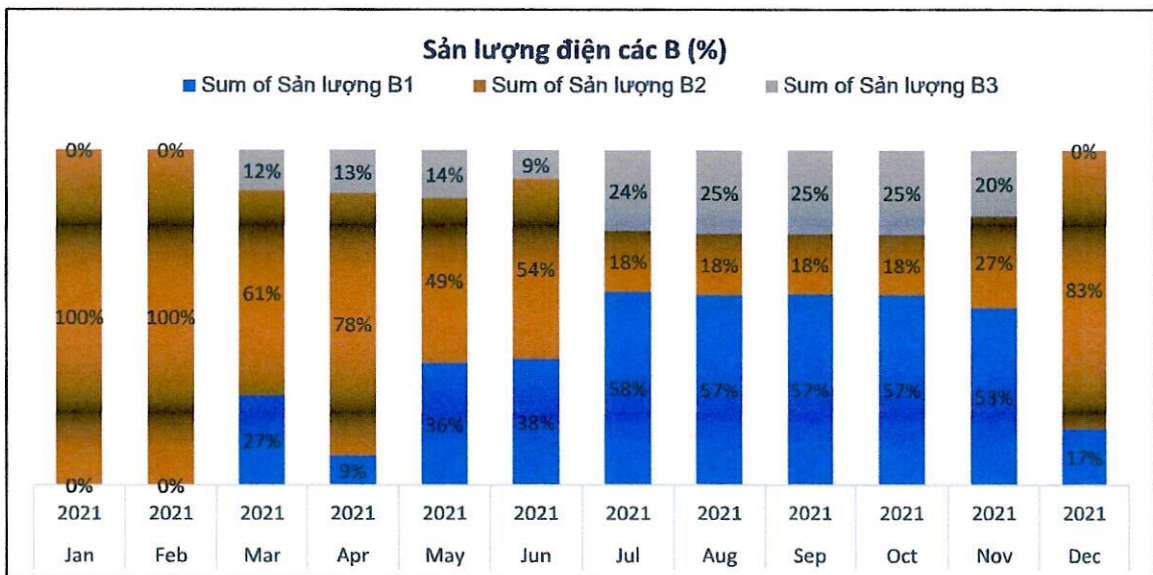
Biểu % giờ phát điện 2021 của NMTĐ Dakglun (Tỷ trọng biểu giá)
