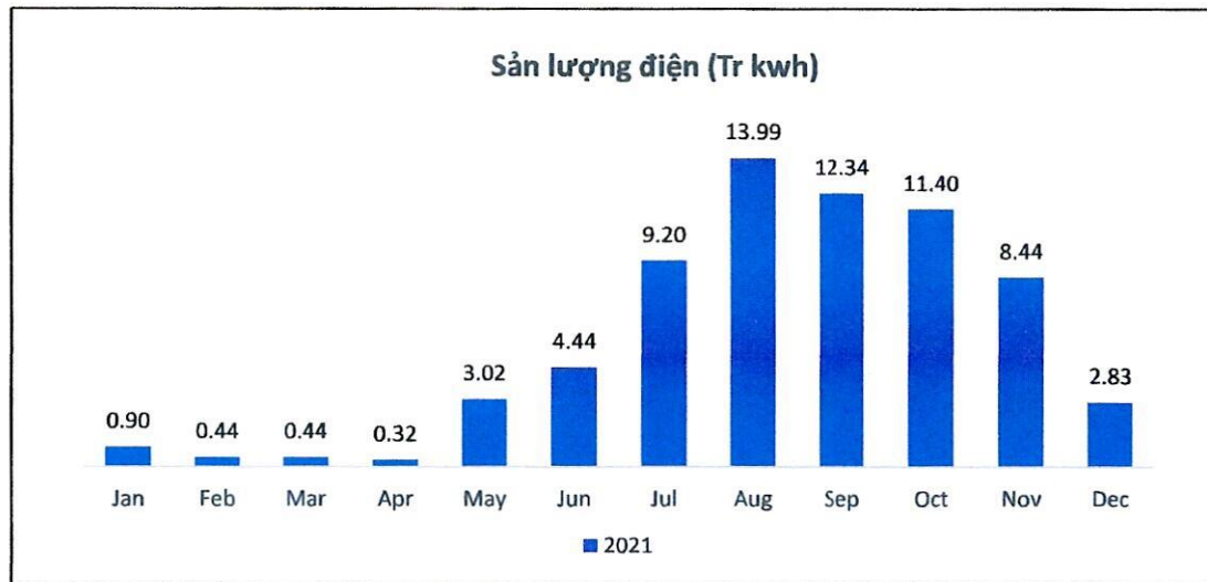
Biểu sản lượng phát điện 2021 của NMTĐ Dakglun
